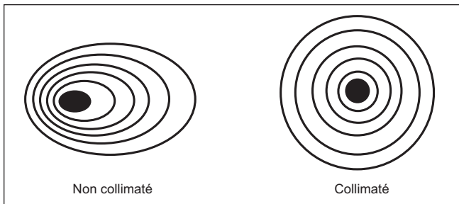
Figure 12. Un test sur une étoile permet de déterminer si les optiques du télescope sont correctement collimatées. Une image non mise au point d'une étoile lumineuse à travers l'oculaire doit apparaître comme illustré à droite si les optiques sont parfaitement collimatées. Si le cercle est asymétrique, comme sur la figure de gauche, le télescope doit être collimaté.
