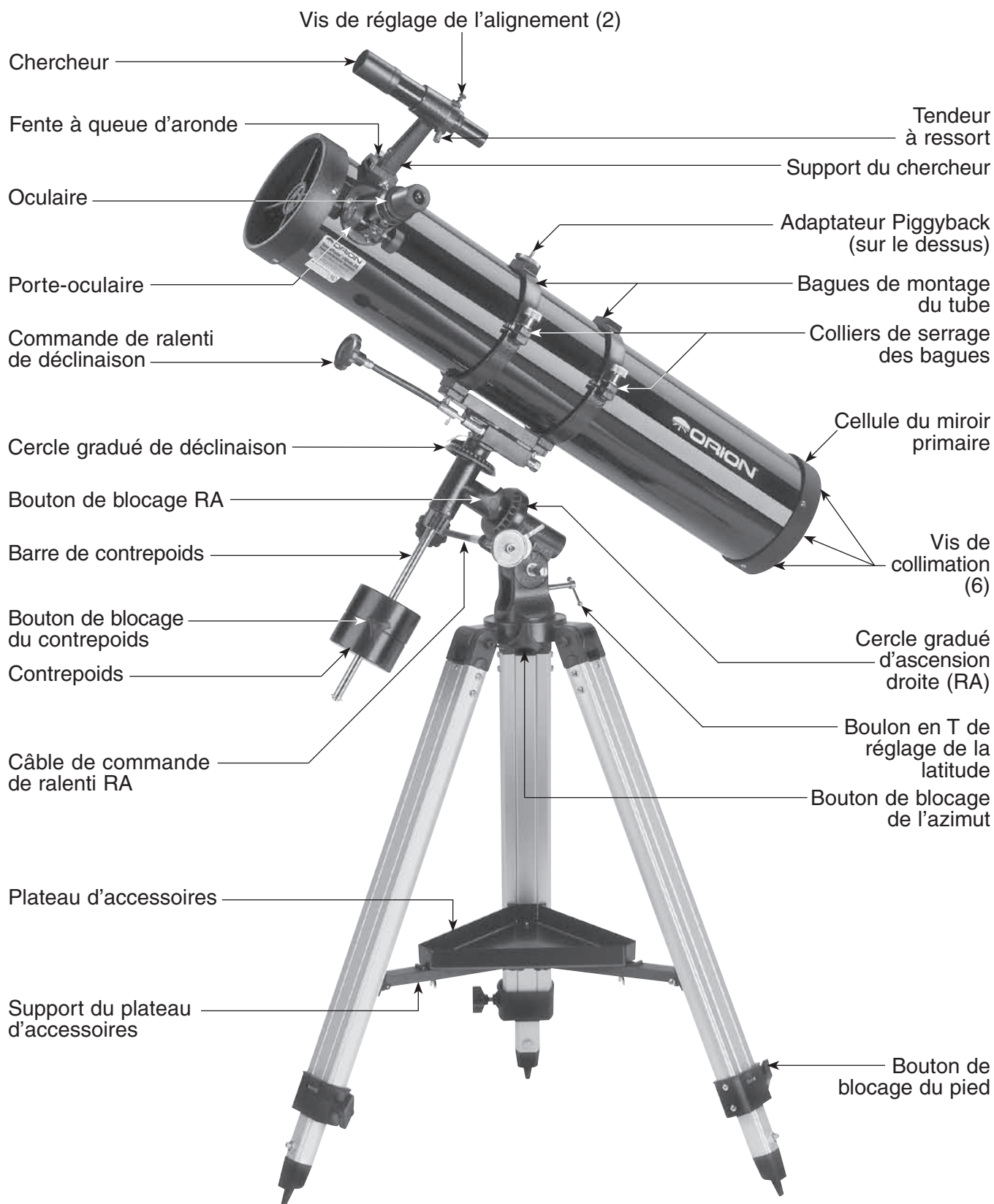
Figure 1. Schéma des pièces du télescope SpaceProbe 130 EQ
