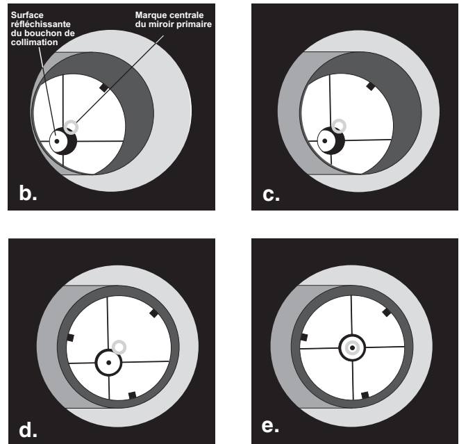
Figure 8. Collimation de l'optique (a) Lorsque les miroirs sont correctement alignés, lorsque vous regardez à travers le tube télescopique du porte-oculaire vous devriez apercevoir quelque chose de semblable à ça. (b) L'œillet de collimation étant en place, la vue peut ressembler à ceci, si l'optique est désalignée. (c) Ici, le miroir secondaire est centré sous le système de mise au point, mais il doit être ajusté (incliné) de manière à ce que le miroir primaire soit visible dans sa totalité. (d) Le miroir secondaire est correctement aligné, mais le miroir primaire doit toujours être ajusté. Lorsque le miroir primaire est correctement aligné, le « point » est centré, comme illustré en (e).
