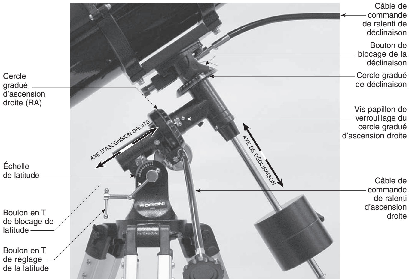
Figure 2. Montage équatoriale du SpaceProbe 130.
