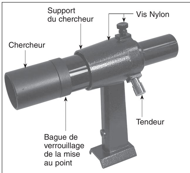
Figure 3a. Le chercheur 6 x 26 à redresseur
