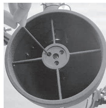
Figure 10. Ajustez l'inclinaison du miroir secondaire en desserrant ou en serrant les trois vis d'alignement à l'aide d'une clé Allen 2 mm
