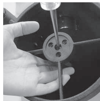
Figure 9. Pour centrer le miroir secondaire sous le porte-oculaire, maintenez le support du miroir en place d'une main tout en ajustant le boulon central à l'aide d'un tournevis cruciforme. Ne touchez surtout pas la surface du miroir !
