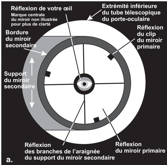
Figure 8. Collimation de l'optique (a) Lorsque les miroirs sont correctement alignés, lorsque vous regardez à travers le tube télescopique du porte-oculaire vous devriez apercevoir quelque chose de semblable à ça. (b) L'œillet de collimation étant en place, la vue peut ressembler à ceci, si l'optique est désalignée. (c) Ici, le miroir secondaire est centré sous le système de mise au point, mais il doit être ajusté (incliné) de manière à ce que le miroir primaire soit visible dans sa totalité. (d) Le miroir secondaire est correctement aligné, mais le miroir primaire doit toujours être ajusté. Lorsque le miroir primaire est correctement aligné, le « point » est centré, comme illustré en (e).
