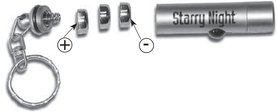
Figura 1. El lado positivo (+) de las tres pilas debe mirar hacia el extremo del llavero (o parte posterior) de la linterna y el negativo (-) debe mirar hacia el extremo del LED (o parte delantera) de la linterna.
